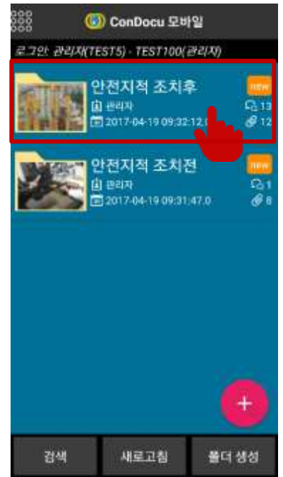
- 폴더 선택
